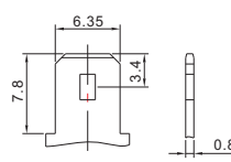
F2 Terminal
